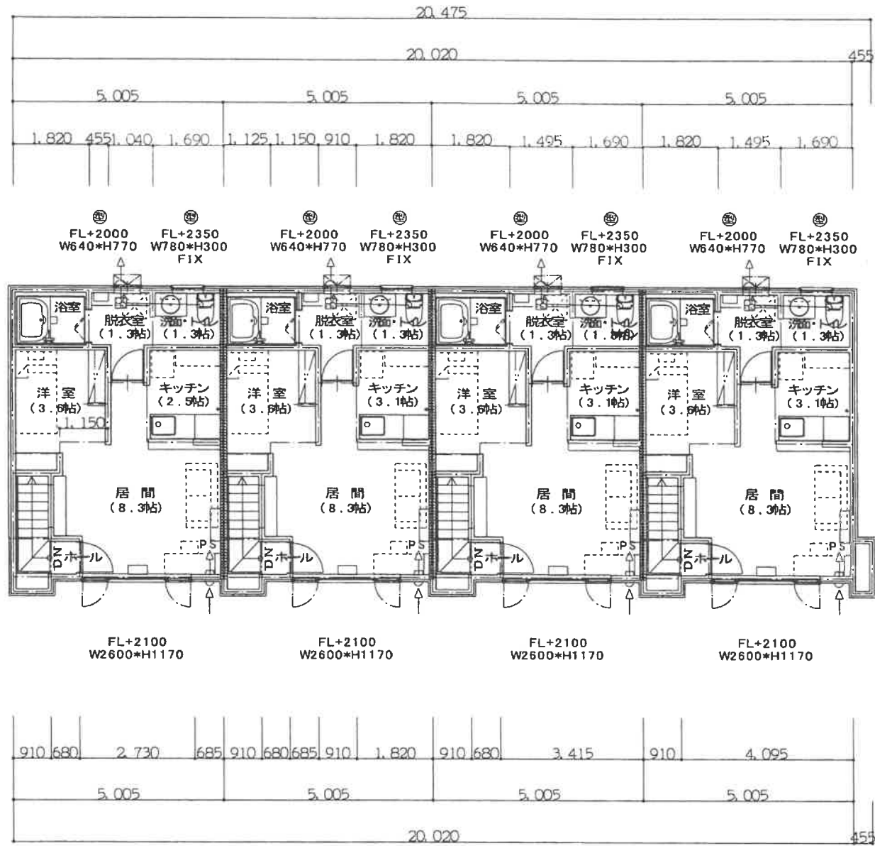
2階平面図 SCALE 1 : 100
